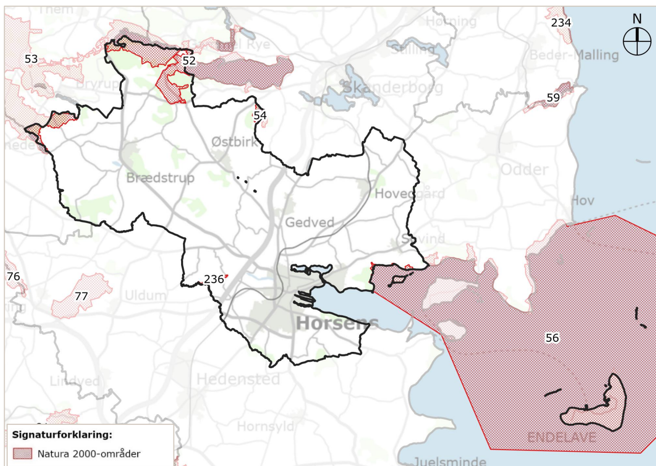
Figur 3-1: Natura 2000-områder (Miljøstyrelsen, 2020).
