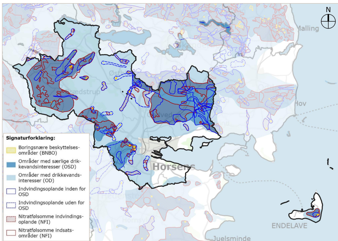
Figur 3-2: Grundvandsinteresser og -beskyttelse (Miljøstyrelsen, 2020).
